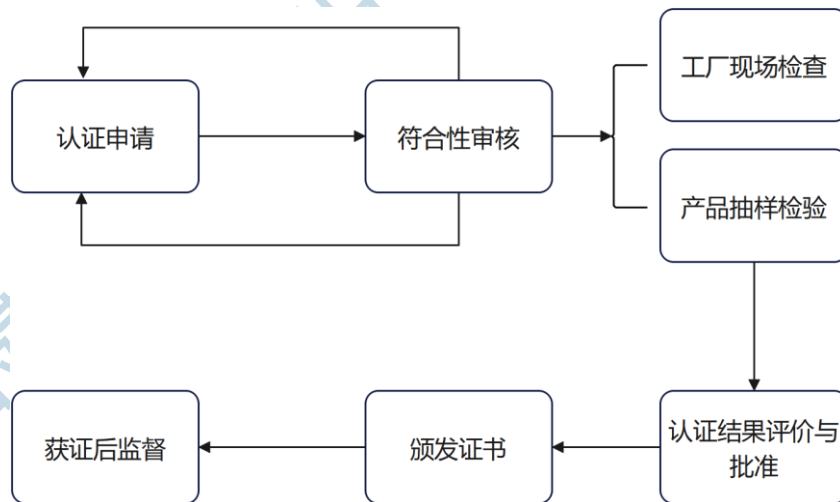
图 1 水泥产品碱含量限值认证流程
